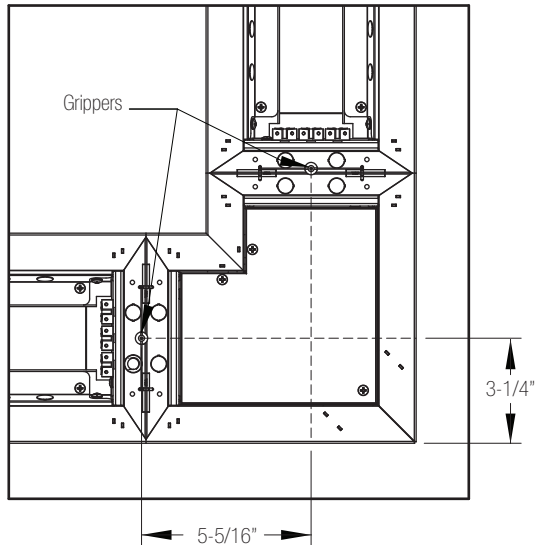
Linero 6 L Corner
